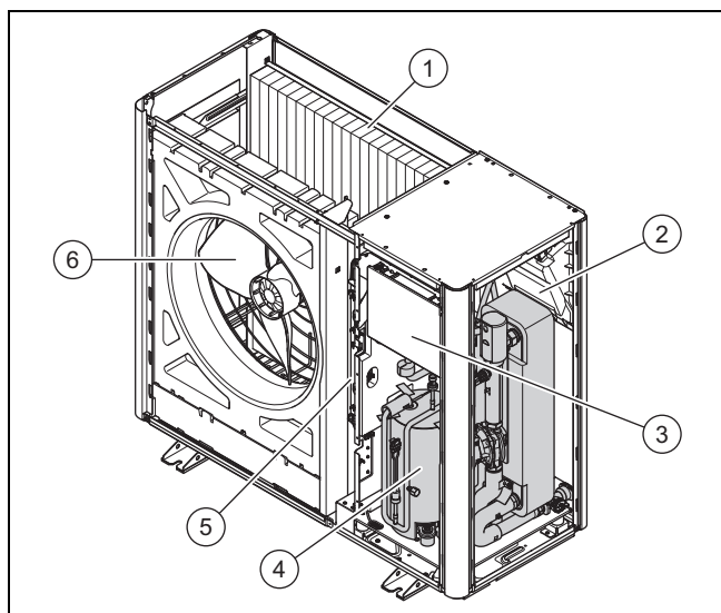
1 Iztvaikotājs 2 Iespējā plate INSTALLER BOARD 3 Iespējā plate HMU 4 Kompresora grupa 5 Grupa INVERTER 6 Ventilators
