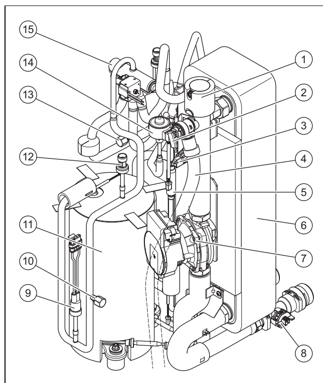
1 Ātrais atgaisotājs 2 Drošības vārsts 3 Apkures kontūra spiediena sensors 4 Noteces šļūtene, drošības vārsts 5 Filtrs 6 Kondensators 7 Apkures sūkņi 8 Caurplūdes sensors 9 Spiediena kontrolierīce augstspiediena zonā 10 Apkopes pieslēgums augstspiediena zonā 11 Kompresors 12 Spiediena sensors augstspiediena zonā 13 Apkopes pieslēgums zema spiediena zonā 14 Elektroniskais izplešanās vārsts 15 4 virzienu pārslēgvārsts
