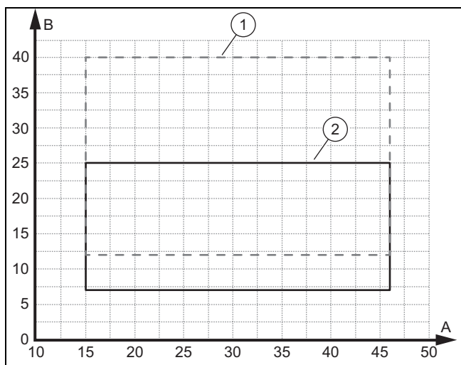
A Välitemperatuur B Küttevee temperatuur 1 Kasutuspiirid, käivitumine, jahutus 2 Kasutuspiirid, jahutuse tavarežiim
