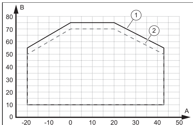
A Välitemperatuur B Küttevee temperatuur 1 Kasutuspiirid, tavarežiim, soe vesi 2 Kasutuspiirid, käivitumine, soe vesi
