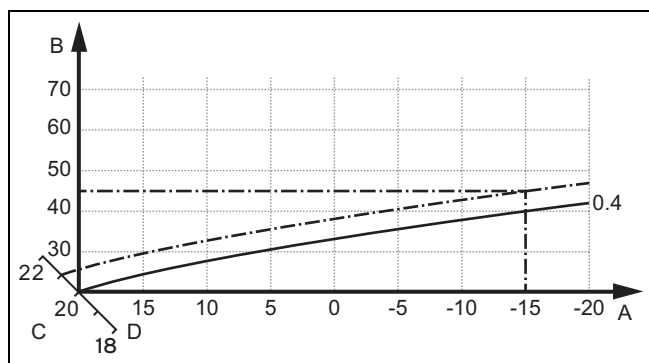
A Lauko temperatūra, °C B Tiekiamojo srauto temperatūra, °C C Patalpos nustatytoji temperatūra, °C D a ašis
